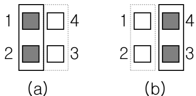
FigureC-11 JP9 Configuration
